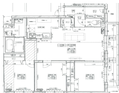
1号室 (3LDK)
